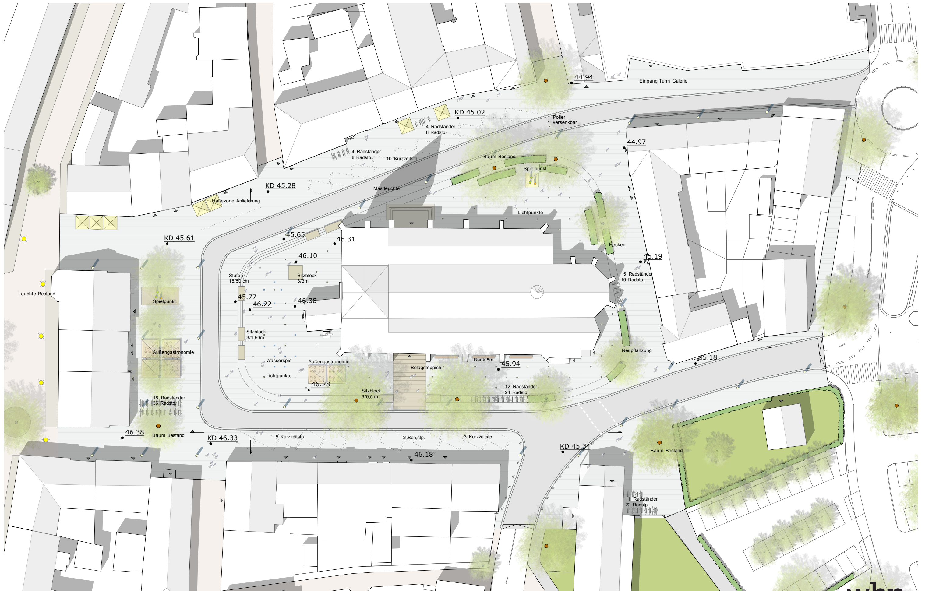
26.06.2013 Lageplan Variante B Schrägstellplätze 30Grad beidseitig 1:500
